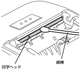
印字ヘッド
